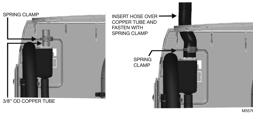
Fig. 11. Condensate return.
